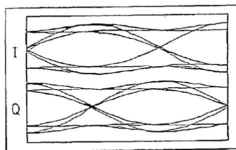
FQPSK-B MEAS.
