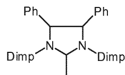
(IIIr)
