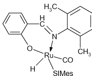
(1a)-SIMes
