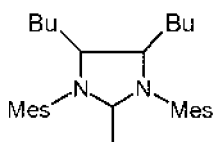
(IIIle)
