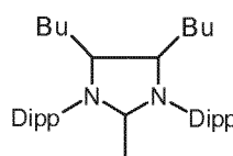
(III m)
