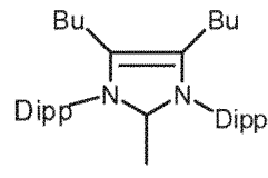
(IIIln)
