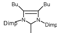
(III u)
