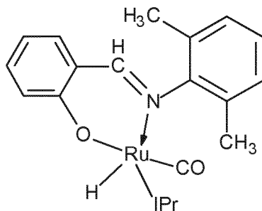
(1a)-IPr
