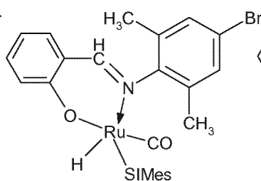
(1b)-SIMes
