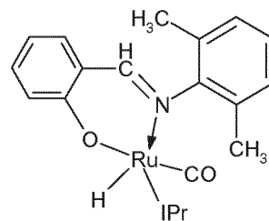
(Ia)-IPr
