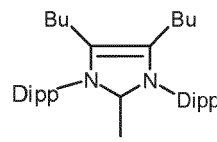
(III m)
