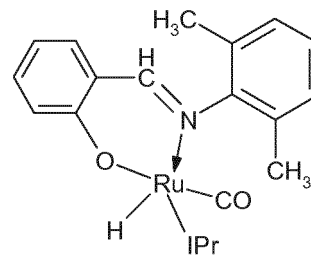
(1a)-IPr
