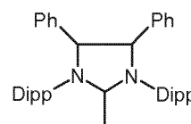
(III j)
