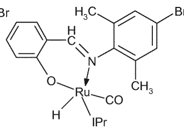
(1b)-IPr
