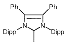
(III k)
