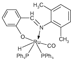
(3a)-PPh 3
