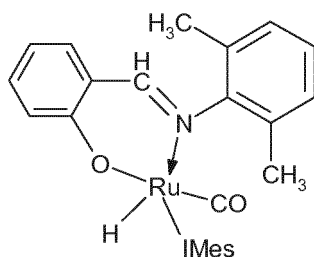
(1a)-IMes
