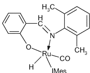
(Ia)-IMes
