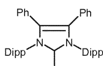
(III k)
