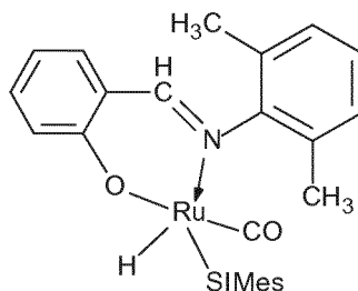
(la)-SiMes
