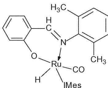
(la)-IMes
