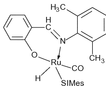
(la)-SIMes
