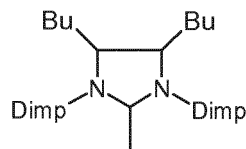
(IIIt)
