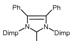
(III s)
