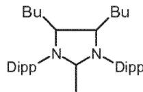
(III l)
