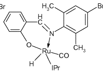
(Ib)-IPr
