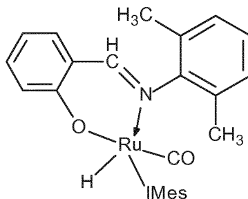
(la)-IMes
