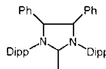
(IIIlj)
