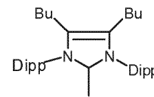
(III n)
