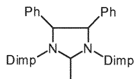
(IIIrr)
