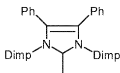
(IIIs)
