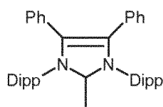
(IIIkk)
