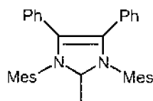
(IIIld)
