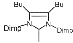
(IIIu)
