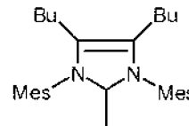
(IIIlf)
