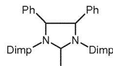
(III r)
