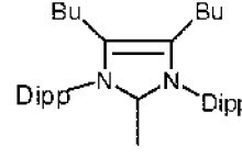
(IIIln)
