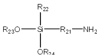
Strukturformel (2)
