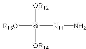
Strukturformel (1)
