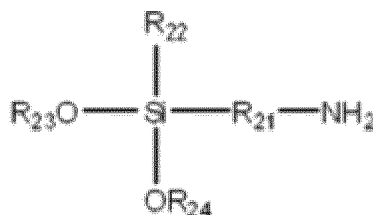
Formules structurale 2
