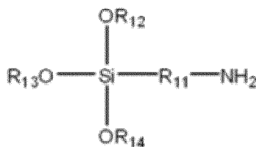
Formule structurale 1
