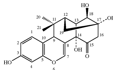
Miroestrol
