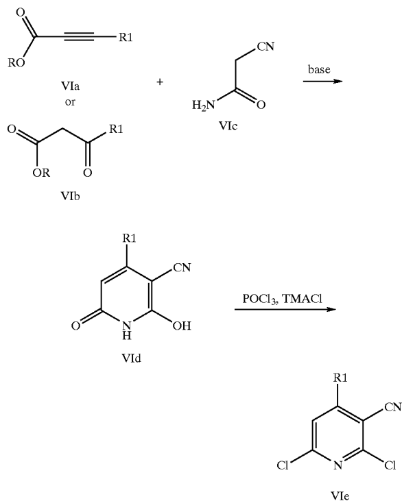
Scheme VI
