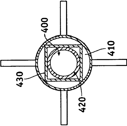
VIEW A-A
