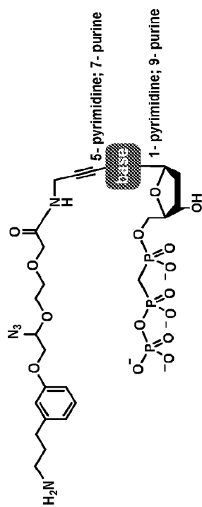
dNTP-PA-Linker 1-NH 2 :
