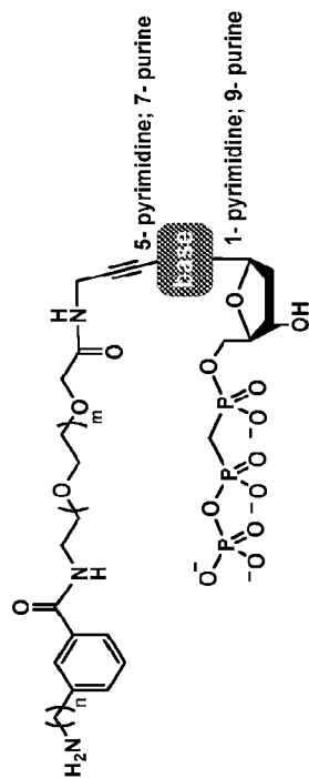
dNTP-PA-Linker 3-NH 2 :
