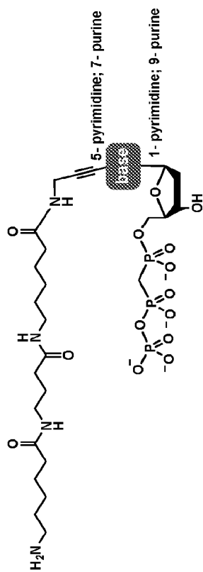
dNTP-PA-N3 Linker-NH 2 :
