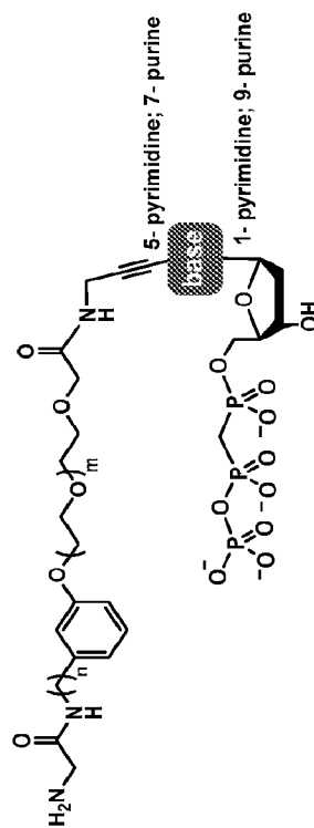
dNTP-PA-Linker 3-NH 2 :
