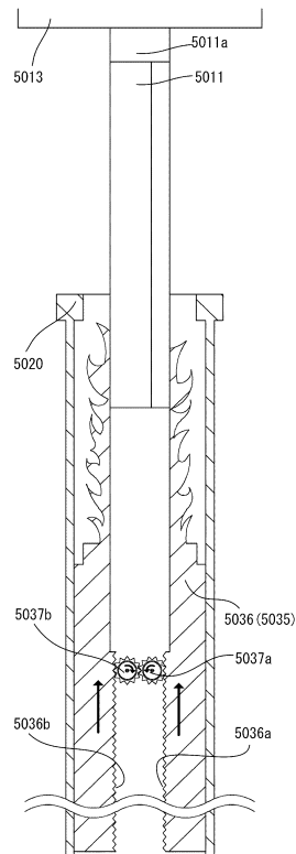
(A) オーラ部材 5035 の完全収容状態
