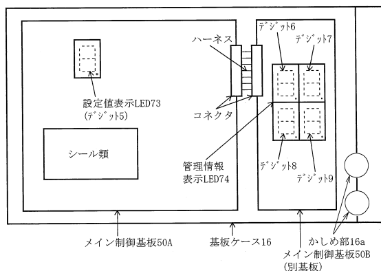
(b) メイン制御基板：例 2
