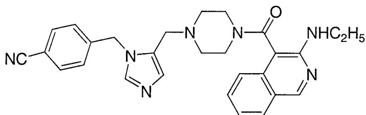
L-452,958
