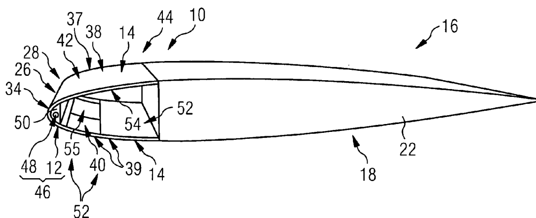
FIG 2 II-II
