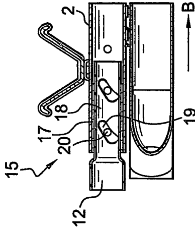
Fig. 8 VY B-B
