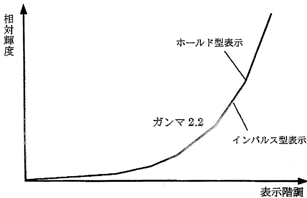
液晶表示装置のガンマ特性
