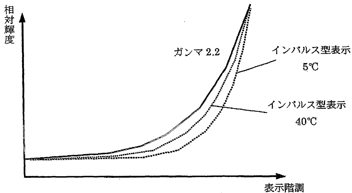
液晶表示装置のガンマ特性
