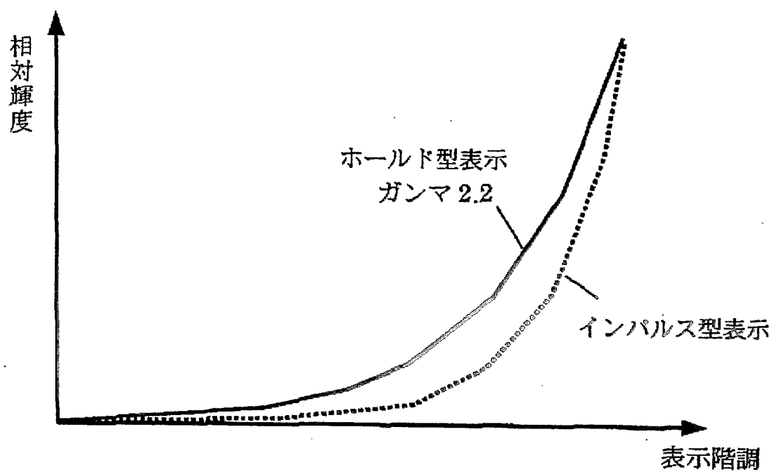
液晶表示装置のガンマ特性
