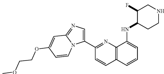
N-(((cis)-3-fluoropiperidin-4-yl)-2-(7-(2-methoxyethoxy)imidazo[1,2-a]pyridin-3-yl)quinolin-8-amine
