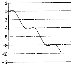
シリーズ 1 m/z トラップ
