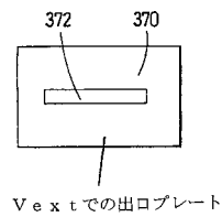
Vextでの出口プレート
