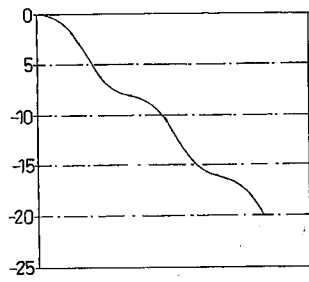
シリーズ 1 m/z 移送
