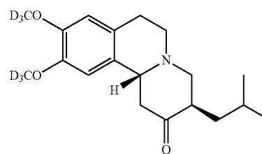
RR-Deutetrabenazine
