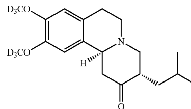
SS-Deutetrabenazine
