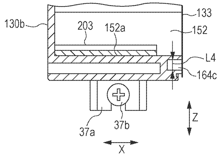
FIG. 20A
