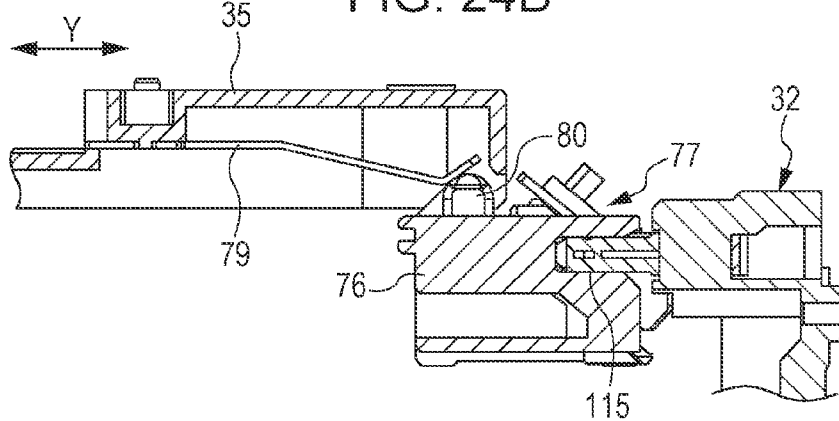
FIG. 24B
