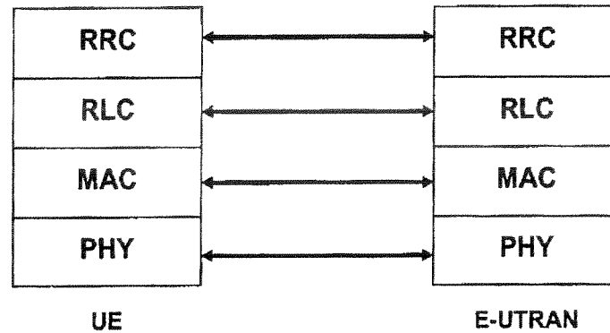
Fig. 3 --Prior Art--
