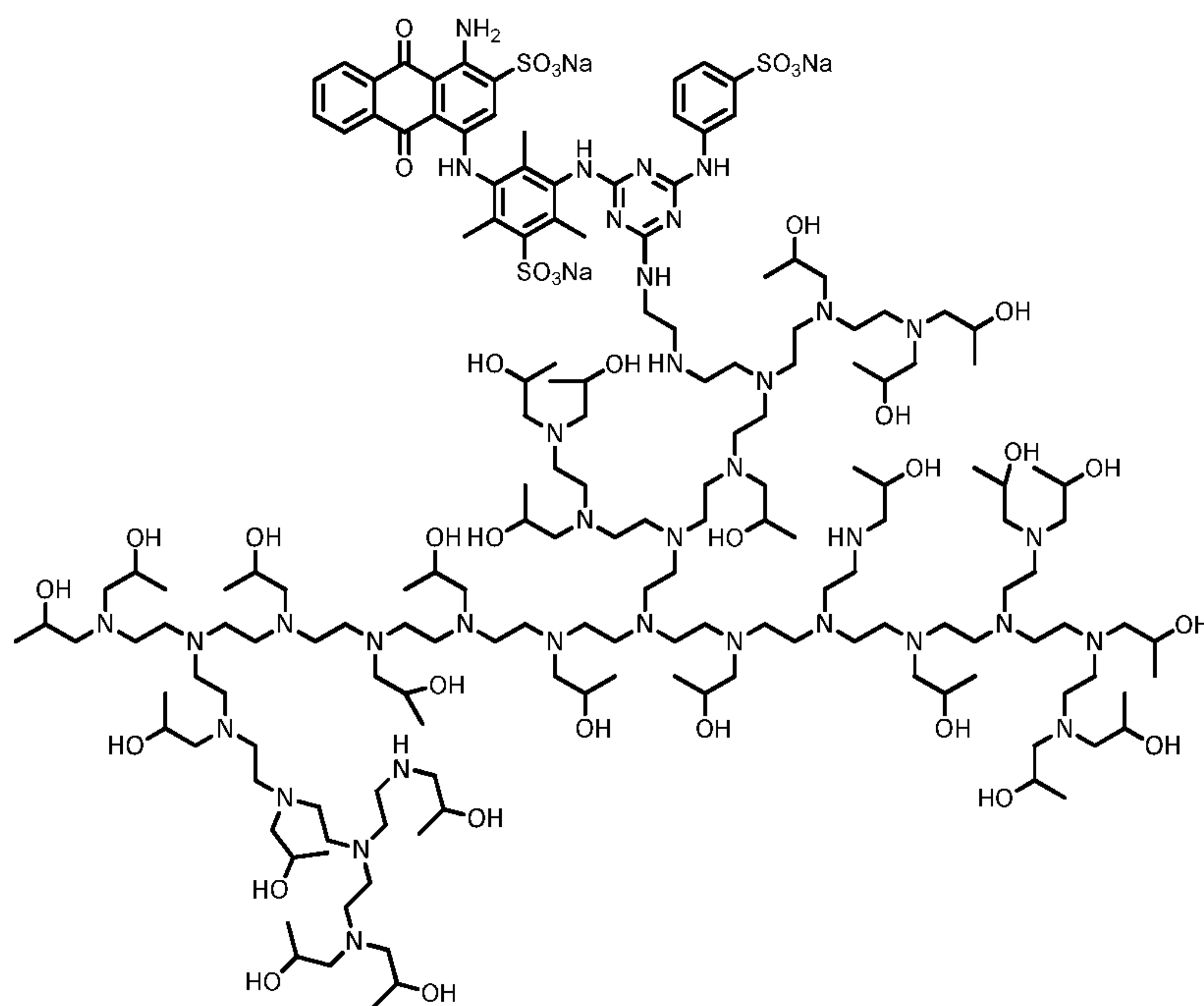
(structure 3).
