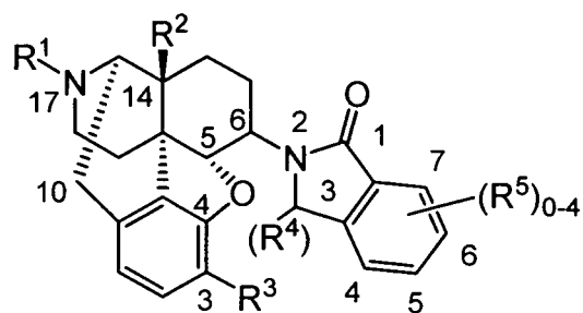
(Ib)
