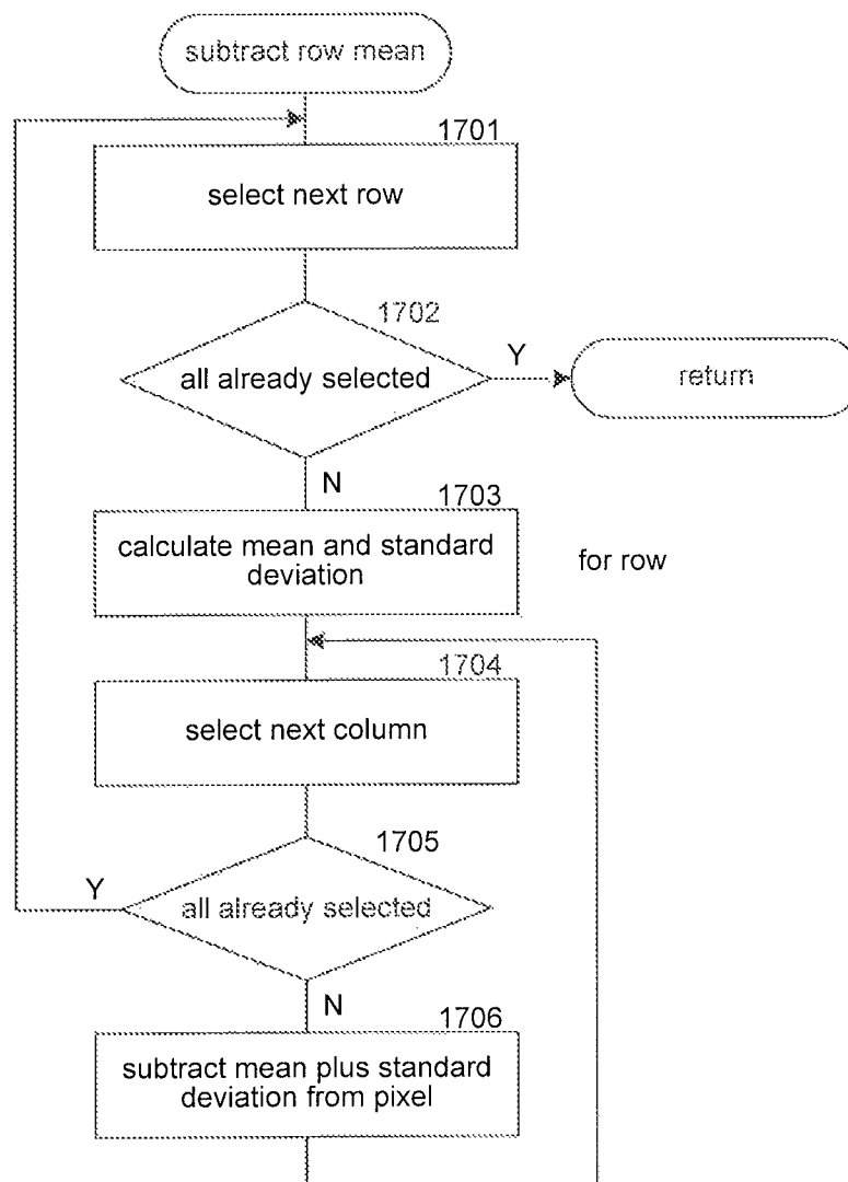
FIG. 17
