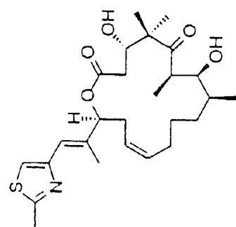
desoxyepothilone A
