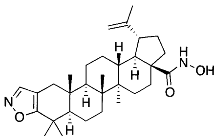
Lup-2-eno[2,3-d]isoxazol-N-hydroxy-28-amide
