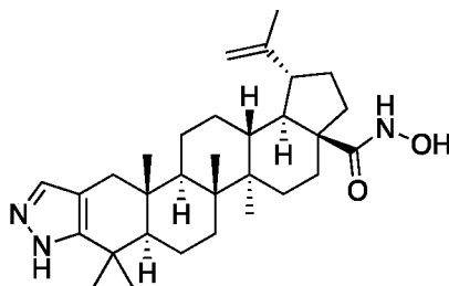
1'H-Lup-20(29)-eno[3,2-c]pyrazol-N-hydroxy-28-amide
