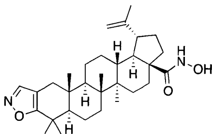
Lup-2-eno[2,3-d]isoxazol-N-hydroxy-28-amide
