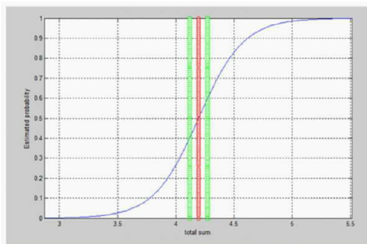
질환군/정상군 판별지표 A7 로지스틱 회귀분석(logistic regression) 결과 (10% 경계영역 설정한 경우)
