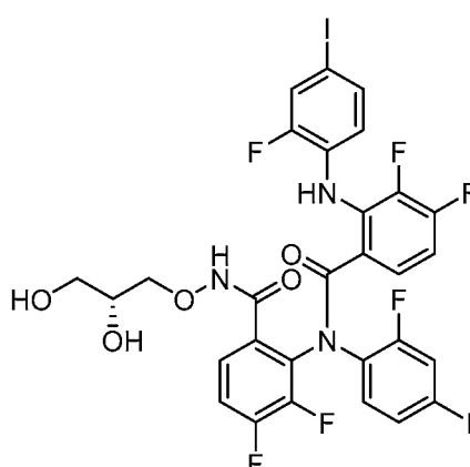
Dimer Exact Mass: 856.93 (d)
