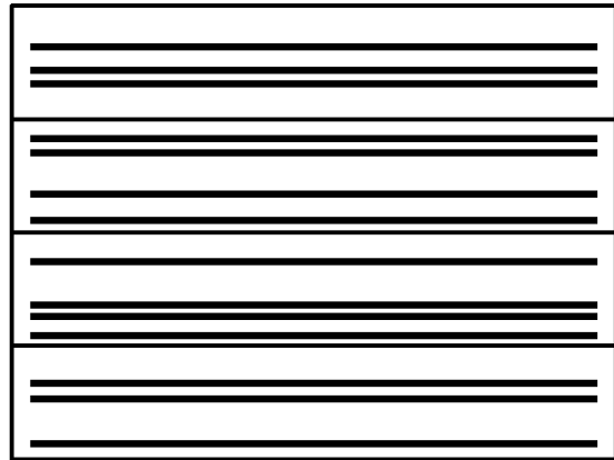
K=2, N_{\text{slab}}=4
