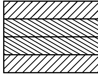
K=2, N_{\text{slab}}=4
