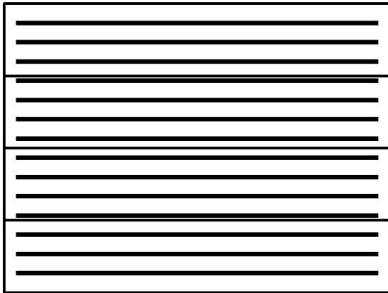
K=2, N_{\text{slab}}=4
