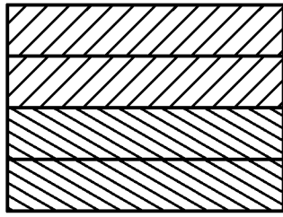
K=2, N_{\text{slab}}=4
