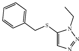
86b 5-(benzylthio)-1-ethyl-1H-1,2,3-triazole
