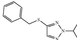
88a 4-(benzylthio)-2-isopropyl-2H-1,2,3-triazole
