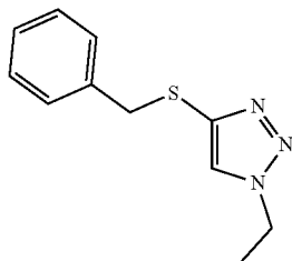
86c 4-(benzylthio)-1-ethyl-1H-1,2,3-triazole
