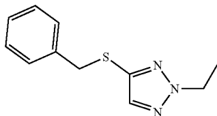
86a 4-(benzylthio)-2-ethyl-2H-1,2,3-triazole
