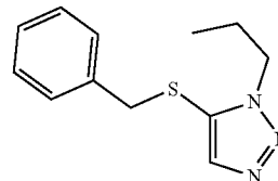
87b 5-(benzylthio)-1-propyl-1H-1,2,3-triazole
