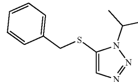
88b 5-(benzylthio)-1-isopropyl-1H-1,2,3-triazole
