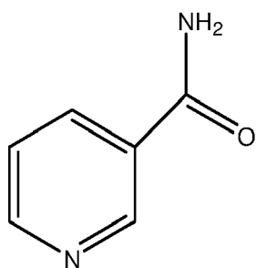
Nicotinamide (NA)
