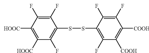
Antifoggant 3
