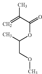
MMEOM monomer
