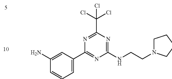
4-(3-aminophenyl)-N-(2-(pyrrolidin-1-yl)ethyl)-6-(trichloromethyl)-1,3,5-triazin-2-amine
