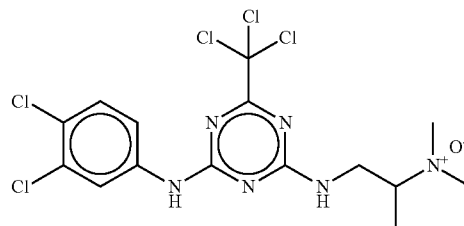
1-((4-((3,4-dichlorophenyl)amino)-6-(trichloromethyl)-1,3,5-triazin-2-yl)amino)-N,N-dimethylpropan-2-amine oxide
