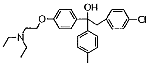
TRIPARANOL
