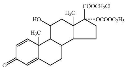
loteprednol etabonate (LE)
