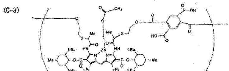
[Chem. 65]
