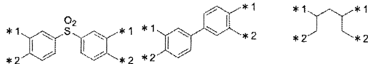
(a-4) Mw 17,000
