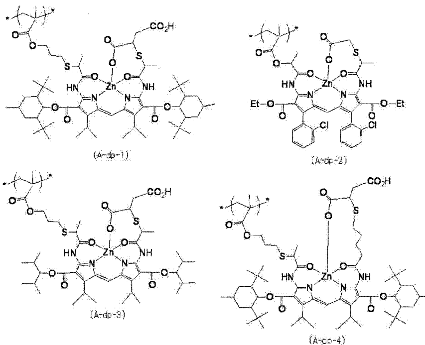
[Chem. 45]
