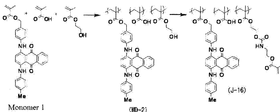
[Chem. 95]
