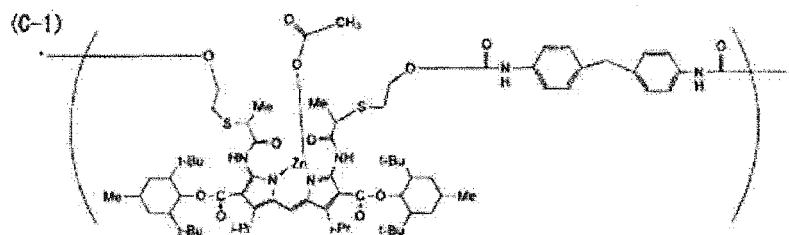
[Chem. 64]
