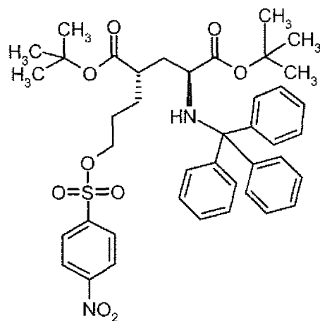
Di-tert-butyl (4S)-4-(3-[[3-nitrophenyl)sulfonyl]oxy]propyl)-N-trityl-L-glutamate
