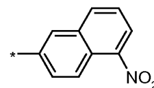
Ij
