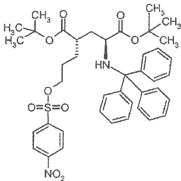
di-tert-butyl (4S)-4-(3-((3-nitrophényl)sulfonyl)oxy)propyl)-N-trityl-L-glutamate
