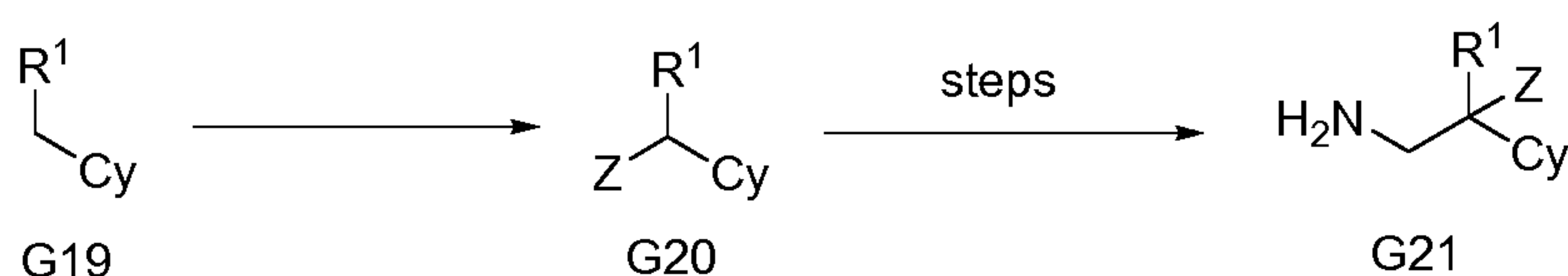
Scheme 9A
