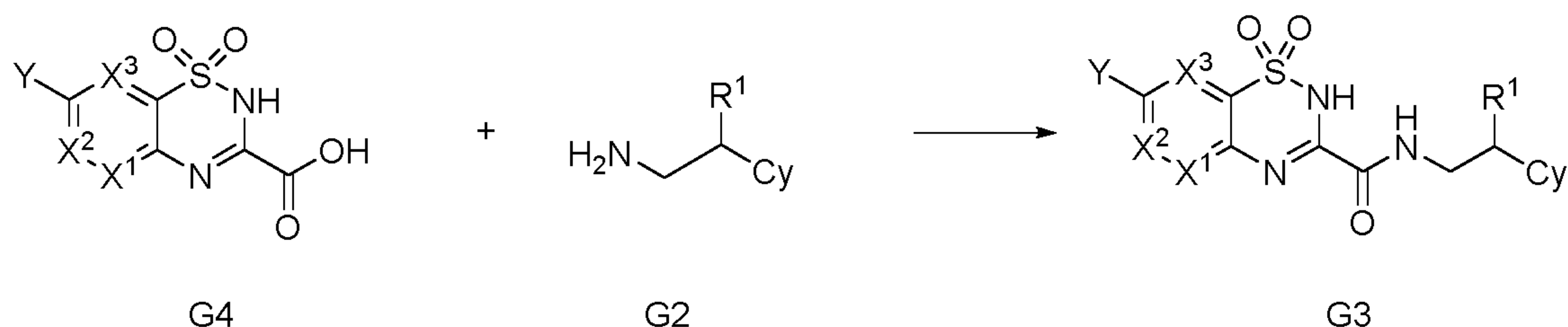
Scheme 2A
