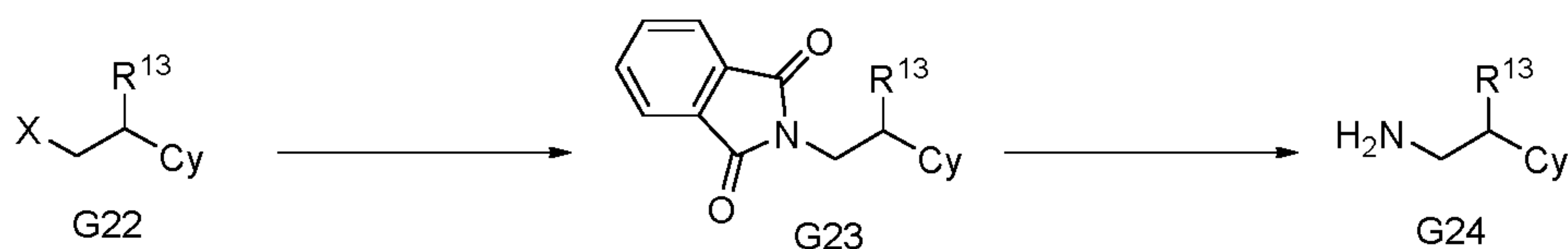
Scheme 10A
