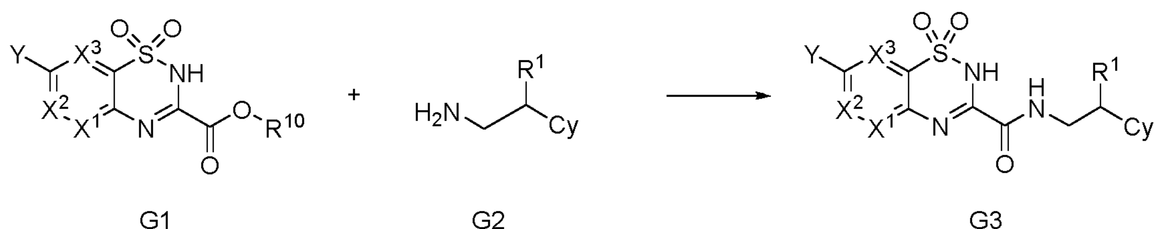
Scheme 1A
