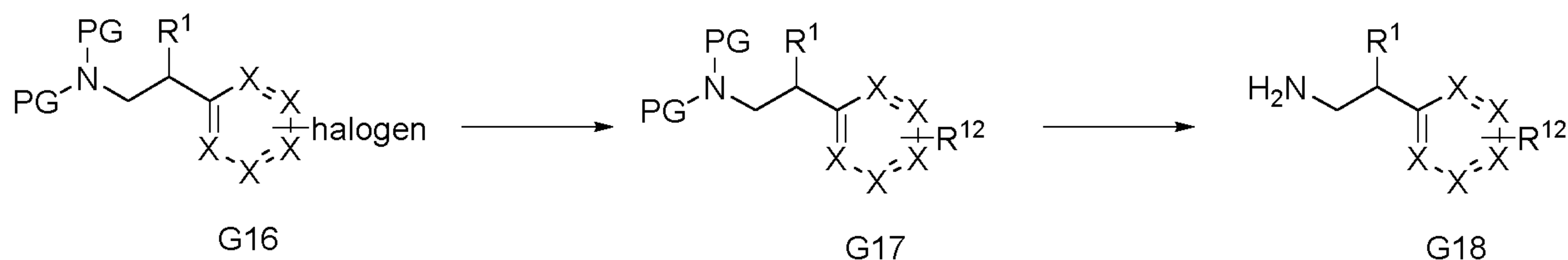
Scheme 8A
