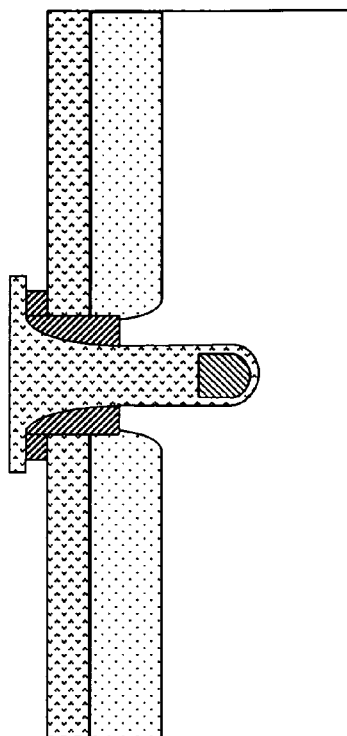
Fig. 23BB'
