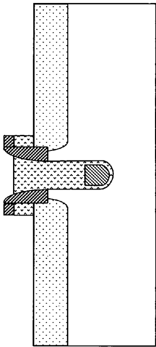
Fig. 26BB'
