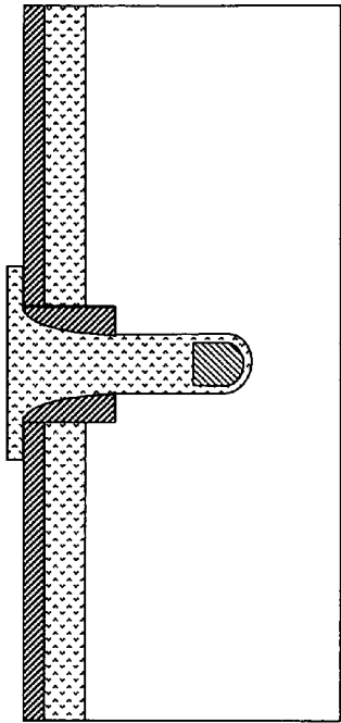
Fig. 20BB'
