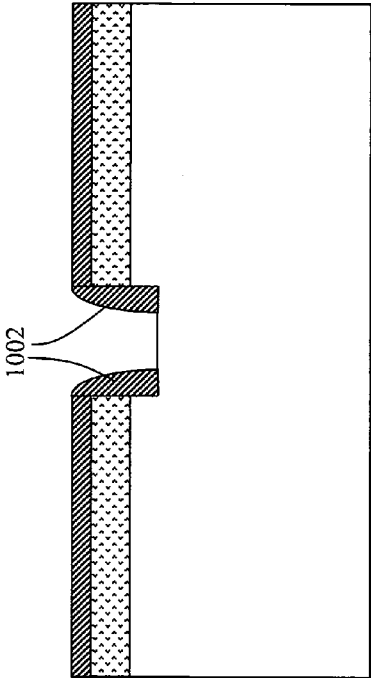
Fig. 10BB'
