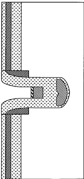
Fig. 24LL'
