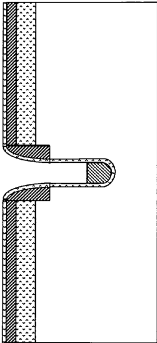
Fig. 14BB'
