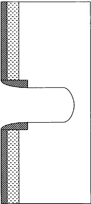
Fig. 11LL'
