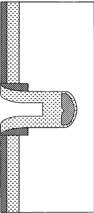
Fig. 16LL'
