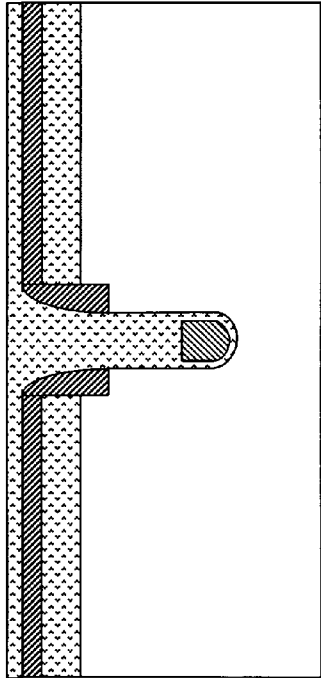
Fig. 17BB'
