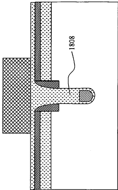
Fig. 18BB'
