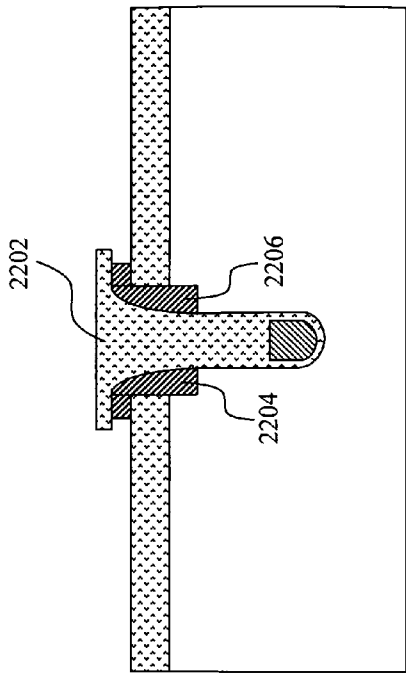
Fig. 22BB'
