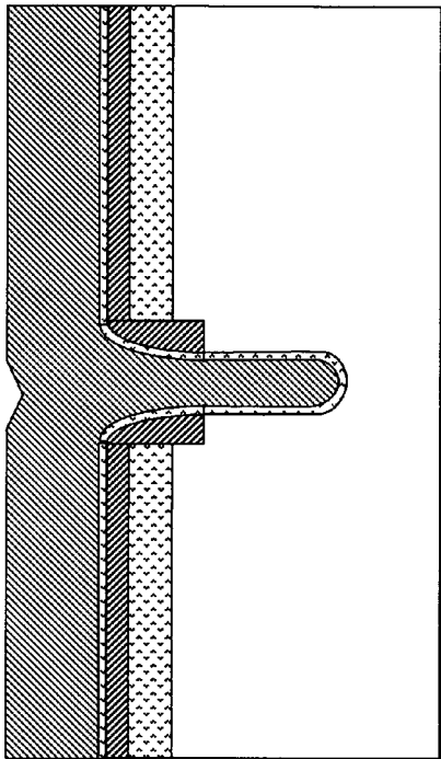
Fig. 13BB'
