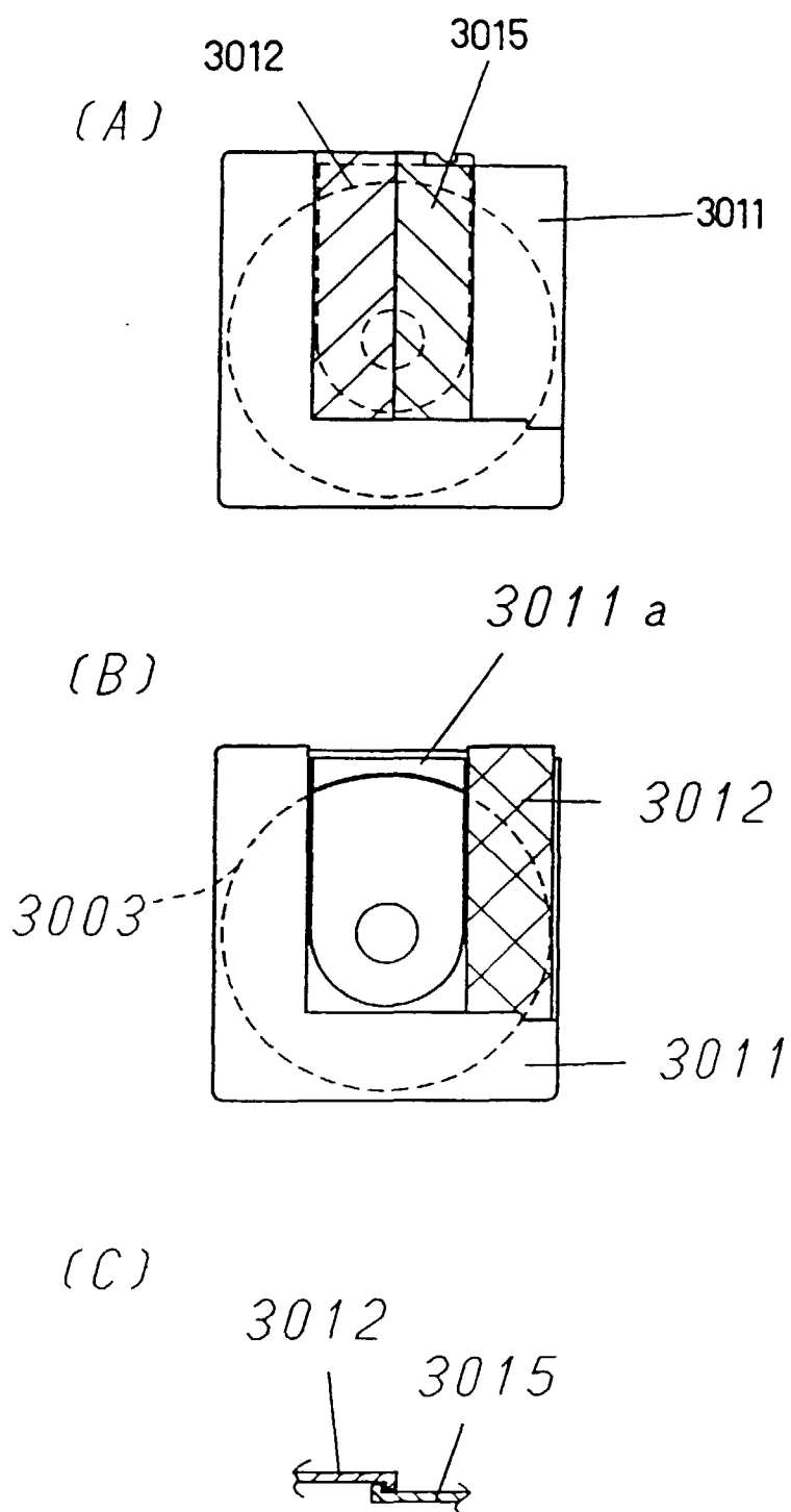
FIG. 65
