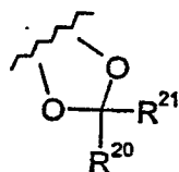
(1.3.1)
