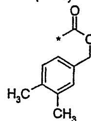
(3.5.10)
