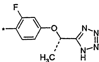
(1.5.16)
