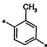
(2.5.41)
