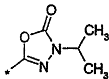
(4.8.30)
