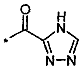
(3.9.10)
