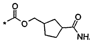
(3.5.13)
