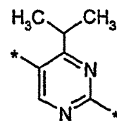
(2.5.16)
