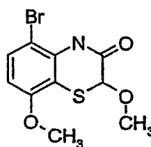
L-651,392
