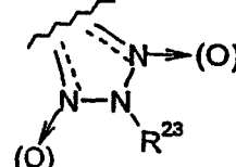
(1.3.15)
