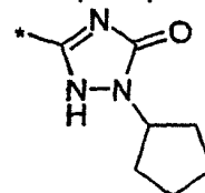
(4.8.12)
