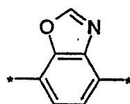
(3.0.42)
