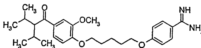
CGS-25019c
