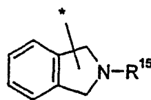
isoindolyl (5.0.3)
