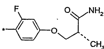
(1.5.29)
