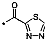
(3.9.17)
