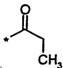
(3.9.1)
