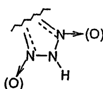
(2.1.18)
