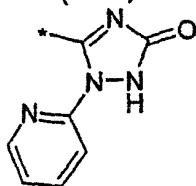
(4.8.13)
