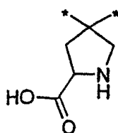
(3.1.28)
