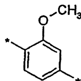
(2.5.6)
