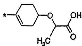
(1.5.32)
