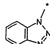
benzotriazolyl (1.4.16)
