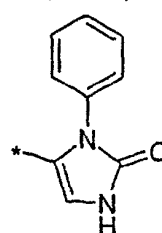
(4.8.27)
