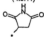
(4.8.48)
