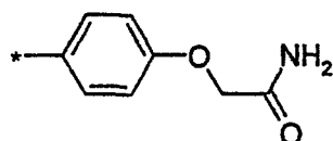
(1.5.11)
