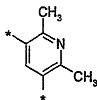
(2.5.15)
