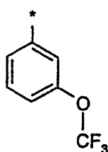
(2.0.10)
