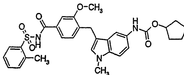
Zafirlukast
