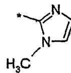
(4.8.16)
