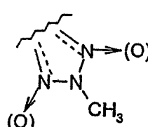
(2.1.19)
