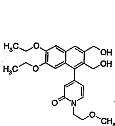
T-440 (0.0.45)
