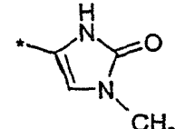
(4.8.24)
