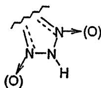
(2.1.18)
