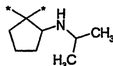
(3.1.13)
