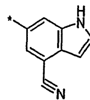
(2.0.63)
