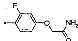
(1.5.12)
