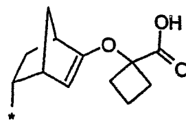
(1.5.33)
