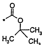
(3.5.15)
