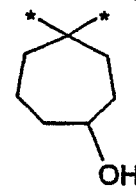
(3.1.19)
