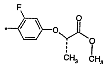
(1.5.18)
