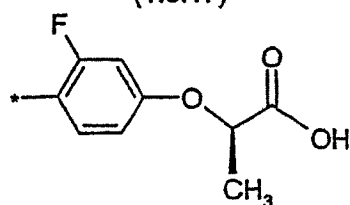
(1.5.20)
