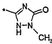
(4.8.10)
