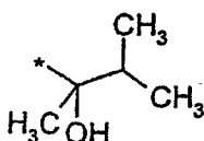
(3.3.3)
