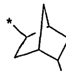
(2.5.28)
