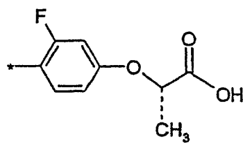
(1.5.17)
