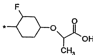
(1.5.26)
