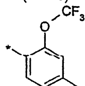
(2.5.39)
