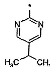
(2.0.32)
