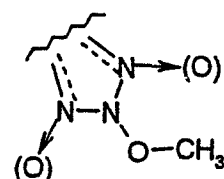
(2.1.20)
