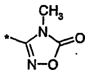
(4.8.34)
