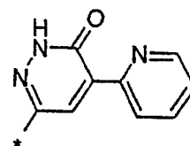
(4.8.64)
