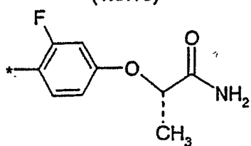
(1.5.19)
