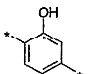
(2.5.37)
