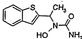
ZYFLO®
