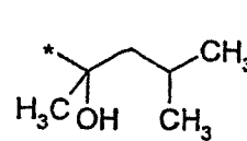
(1.1.7)
