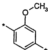
(2.5.6)
