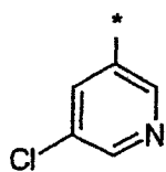
(2.0.29)
