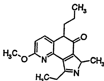
D-22888
