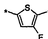
(2.5.48)
