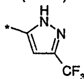
(4.8.47)
