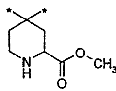
(3.1.30)
