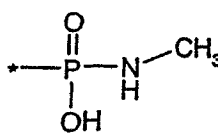
(6.5.2)
