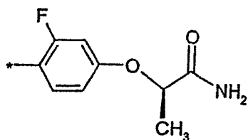
(1.5.22)
