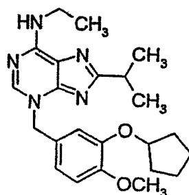
V-11294A (0.0.22)
