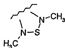
(2.1.16)
