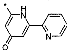
(4.8.58)
