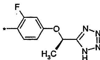
(1.5.14)
