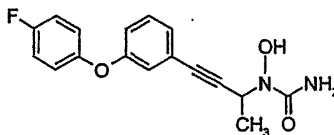
Fenleuton
