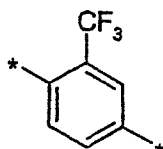
(2.5.7)
