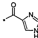
(3.9.13)
