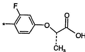
(1.5.17)
