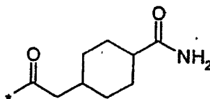
(3.9.7)
