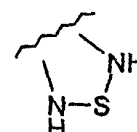
(2.1.6)
