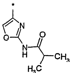
(2.0.37)
