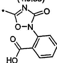
(4.8.42)
