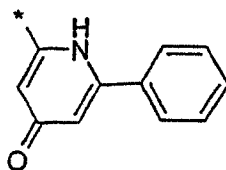
(4.8.57)
