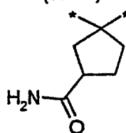
(3.1.11)
