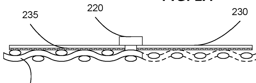
FIG. 2B (A-A')
