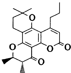
(±)-18a
