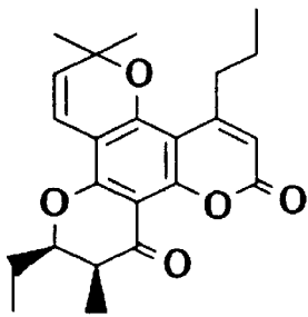
(±)-15d
