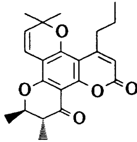
(+)-7
