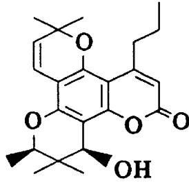
(±)-16a
