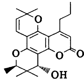
(±)-16b
