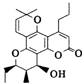
(±)-16h
