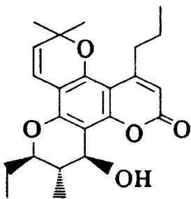
(±)-16f
