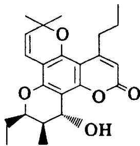
(±)-16g
