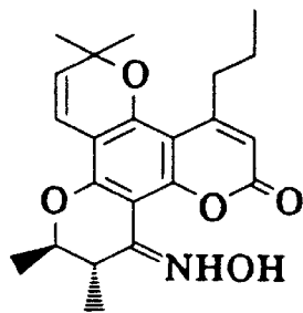
(±)-19a
