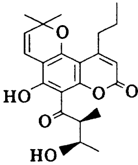
(±)-8a
