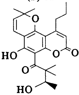
(±)-14a
