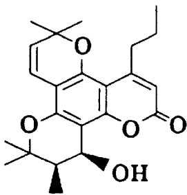
(±)-16c
