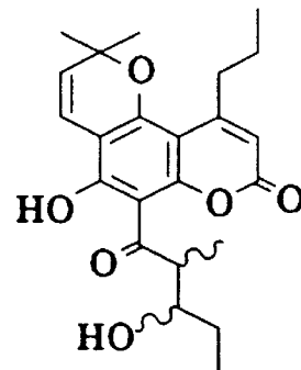
14c
