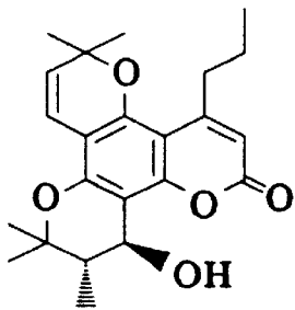
(±)-16d
