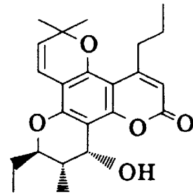
(±)-16b
