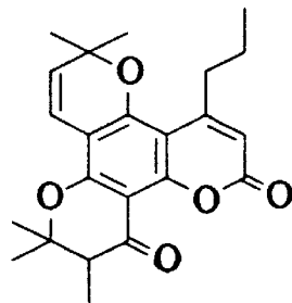
(±)-15b
