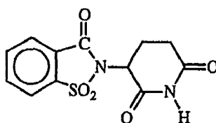
supidimide.
