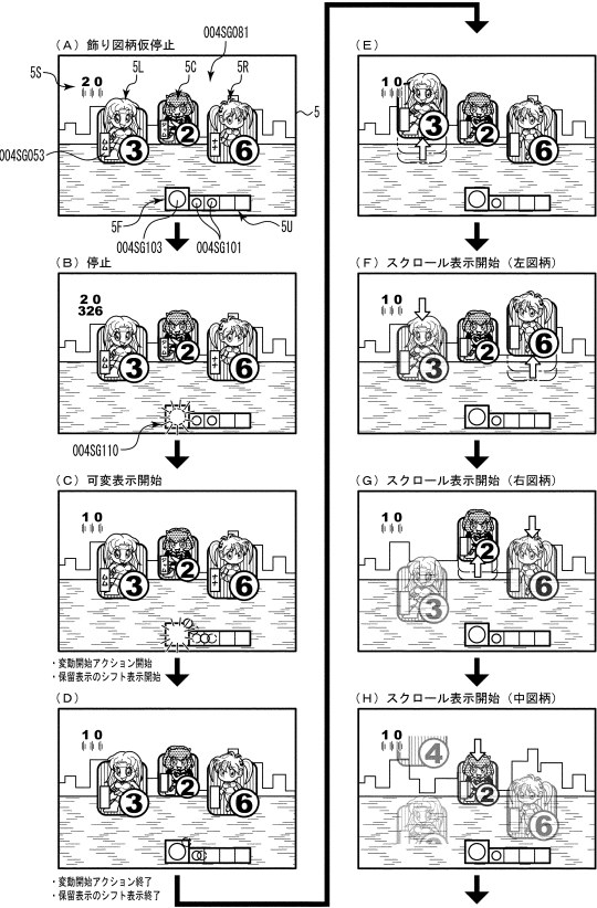
【図12-22】可変表示開始 [第1演出モード]
