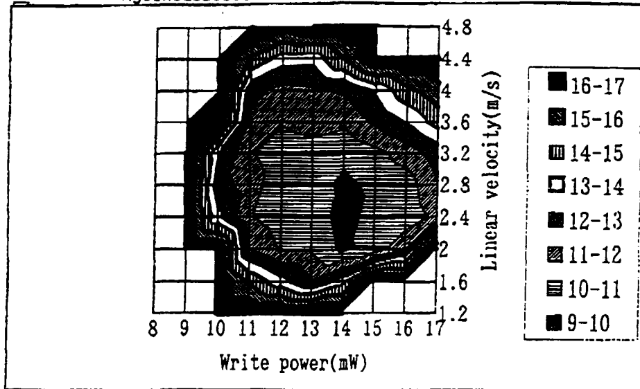
FIGURE 29(b) \text{Ag}_5\text{In}_3\text{Ge}_2\text{Sb}_6\text{Te}_{26}
