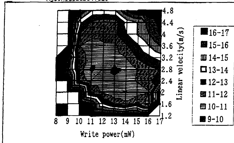
FIGURE 29(b) \text{Ag}_5\text{In}_3\text{Ge}_2\text{Sb}_6\text{Te}_{26}
