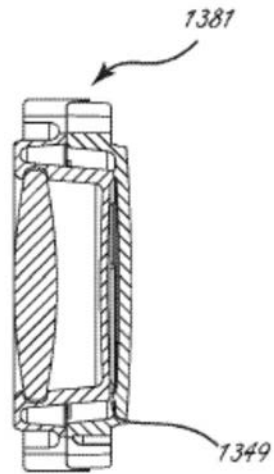
截面B-B
