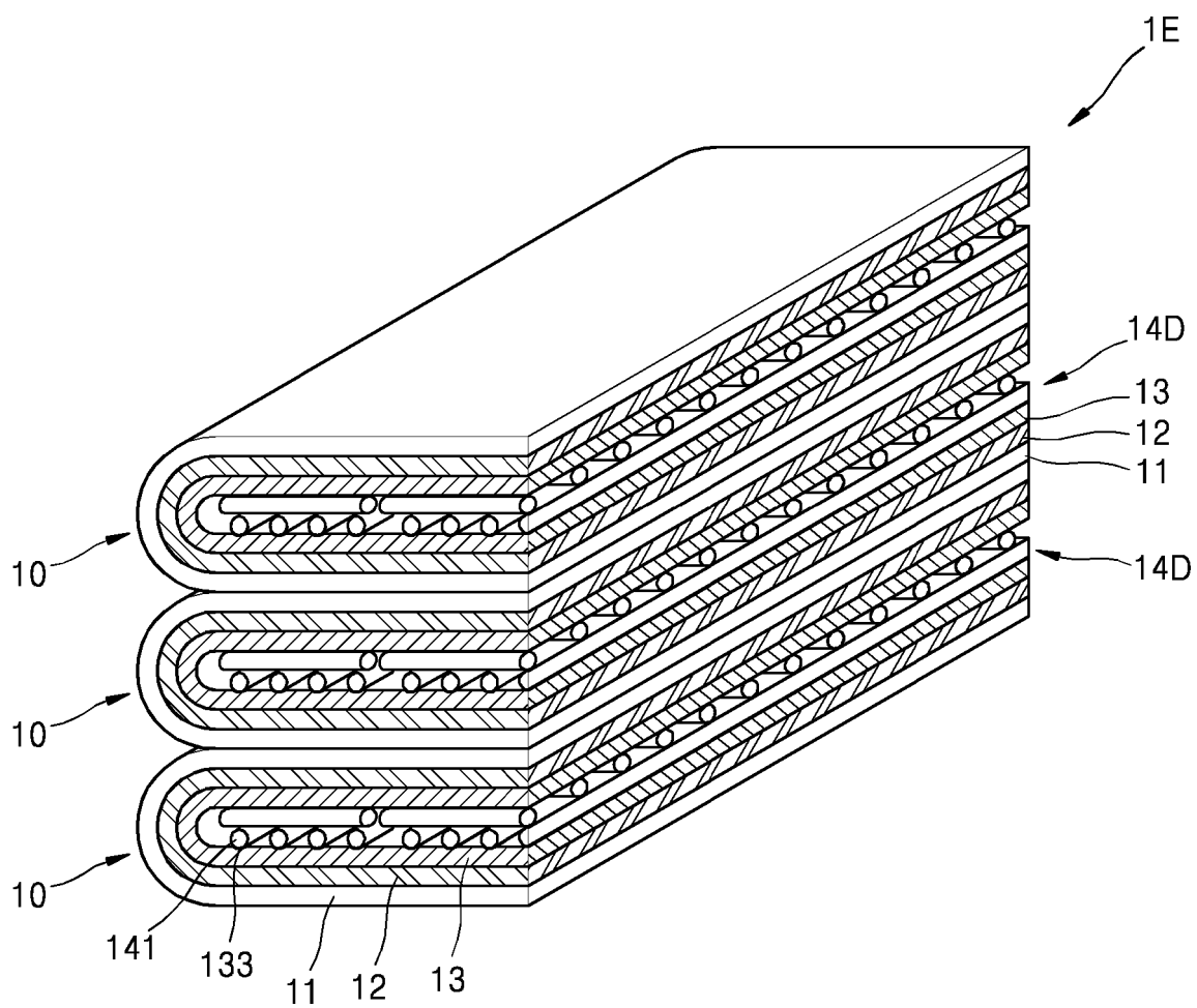
FIG. 11B
