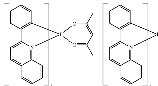
Ir(pq) 2 (acac)
