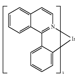
Ir(piq) 3
