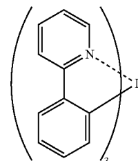
Irppy
