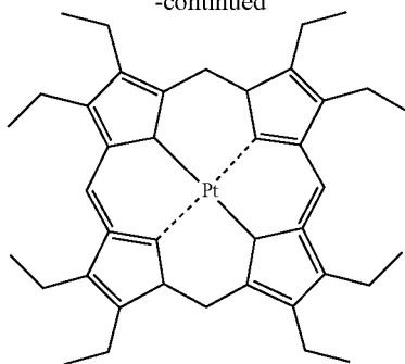
PtOEP
