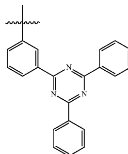
J5
