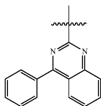
J3
