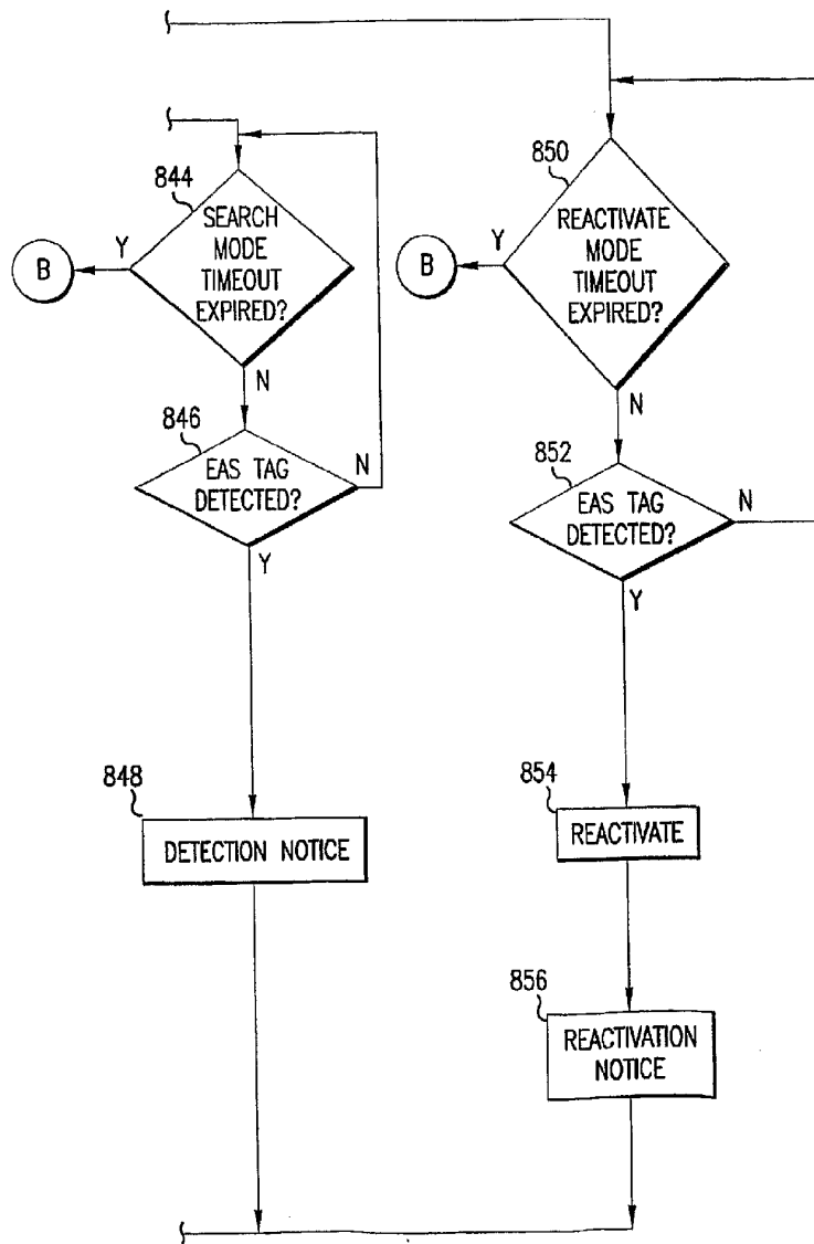
FIG. 8B-2
