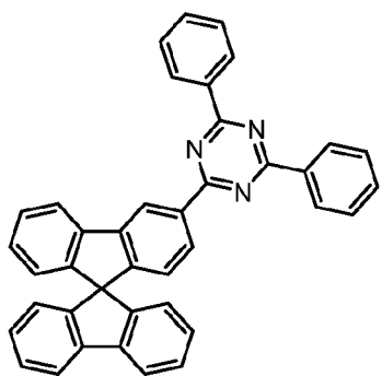
SF3-TRZ
