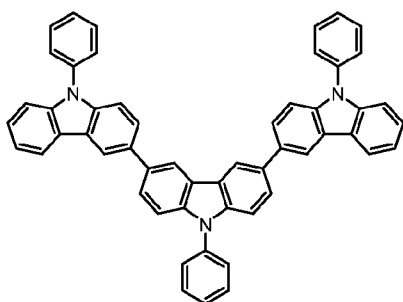
Tris-PCz
