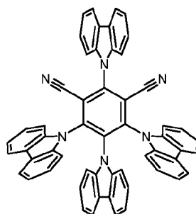
4CzIPN
