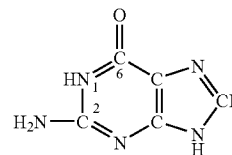
Cosimine (2-amino-6-oxypurine)
